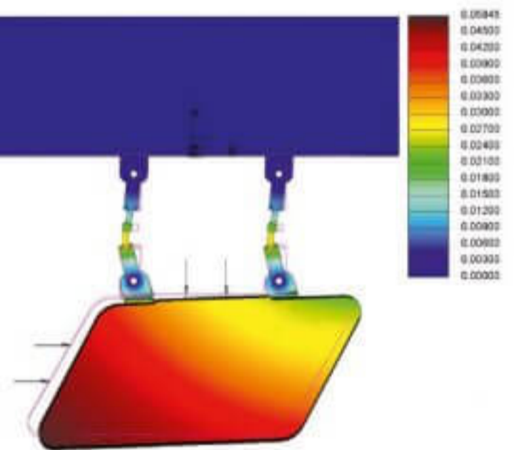
Die Doppelgelenk-Pendelkonstruktion der Aufhängung kann seitliche Windlasten gut aufnehmen.
